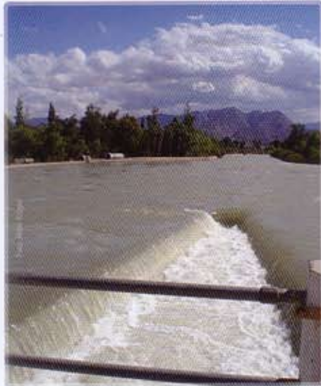
Stausee Ullum (oben) und Bewässerungskanal
